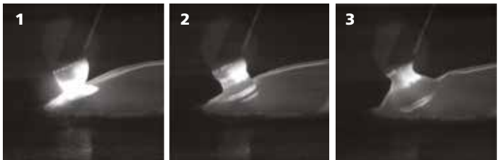
IAC™ – Lodrät fallande svetsning av ett rotsträng i en fjärrvärmelledning. Svetshastigheten ökas betydligt jämfört med traditionell stigande svetsning.
