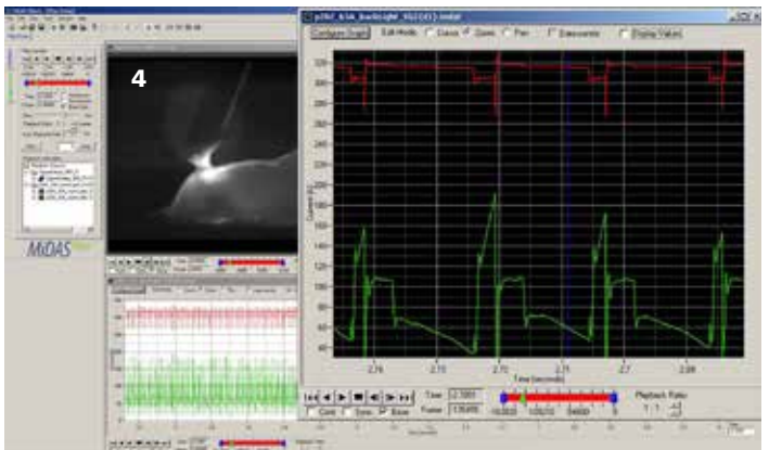
Laborietester i realtid visar full kontroll över IAC-processen även vid dropavgång.
